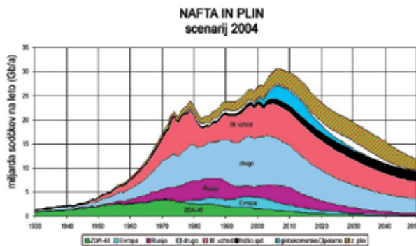
Slika 1.1. Svetovna proizvodnja nafte in vrh proizvodnje. Vir: Novice ASPO
